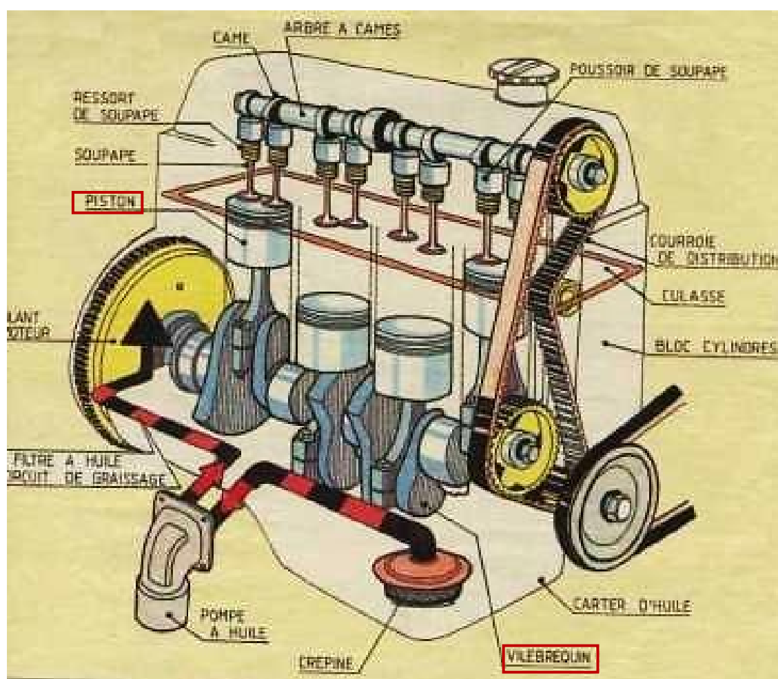
Figure 1: Schéma d'un moteur à 4 temps
