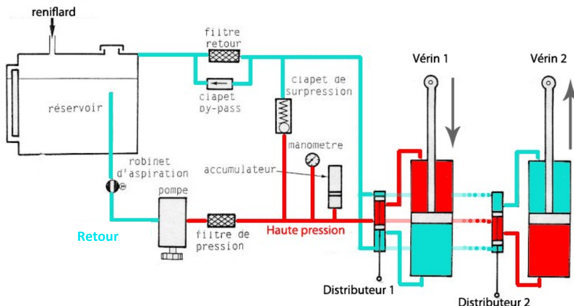
Figure 12: Schéma du circuit hydraulique de tracteur
