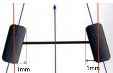
Figure 5 : Réglage du parallélisme (4 RM)
