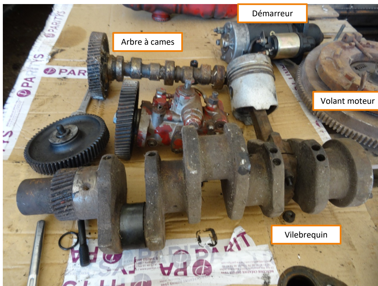
Figure 2: Eléments démontés d'un moteur
