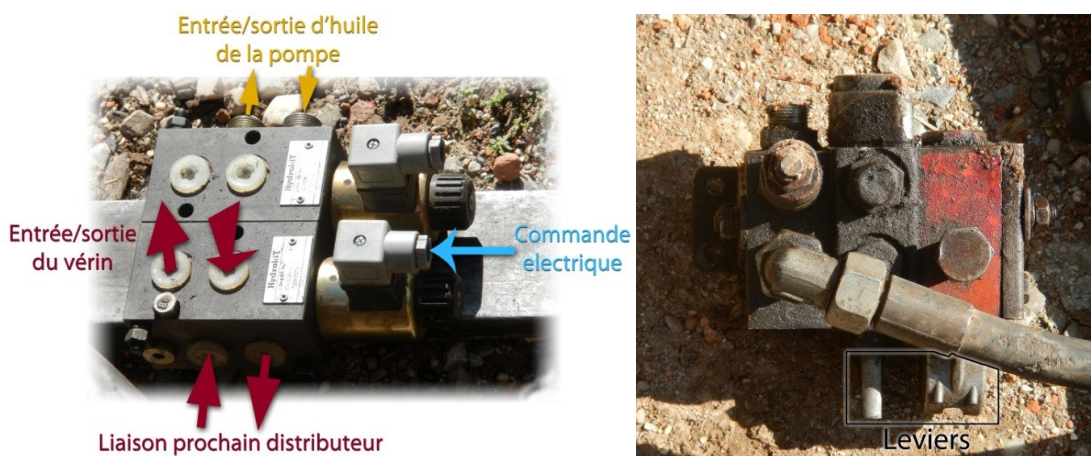
Figure 11: Distributeurs électriques (à gauche) et mécanique (à droite)
