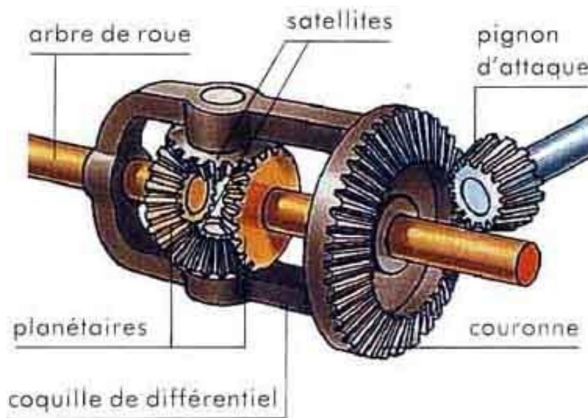
Figure 9: Bloc différentiel
